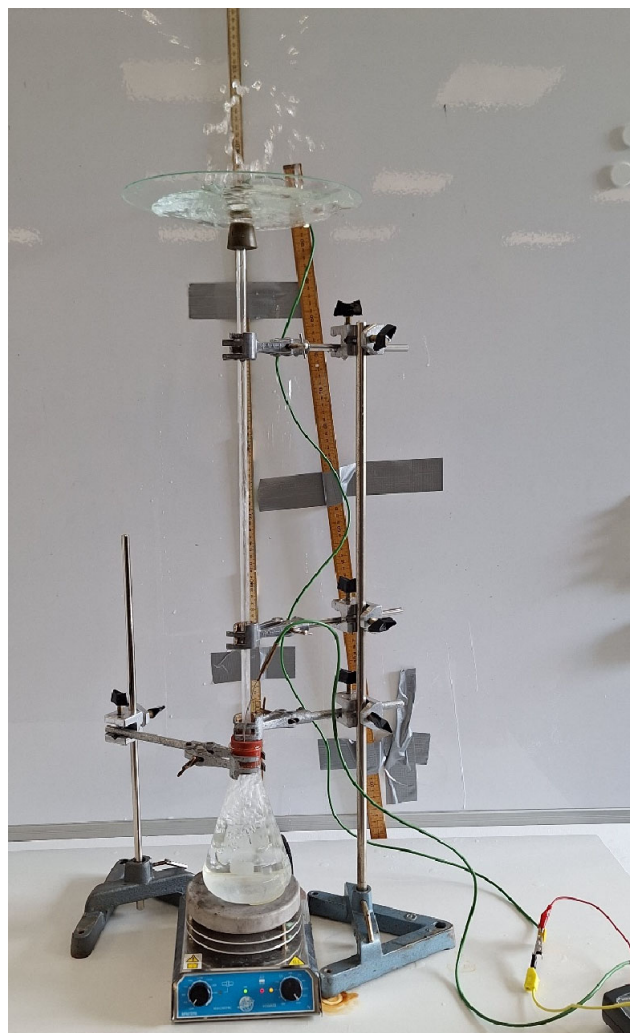
Niko, Maximilian und Niels untersuchen im SoSe24 die Funktionsweise eines Geysirs und optimieren die Auswurfhöhe.
